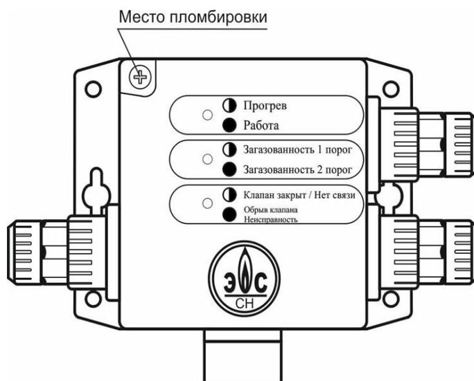
Рисунок 2 - Место пломбировки и нанесения знака поверки в виде оттиска поверительного клейма на корпус сигнализаторов СЗЦ-3-1, СЗЦ-3-2 и их модификаций для ограничения несанкционированного доступа
